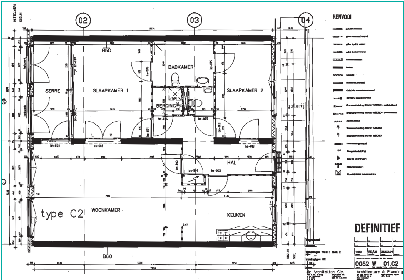
Plattegrond 3-kamerappartement
