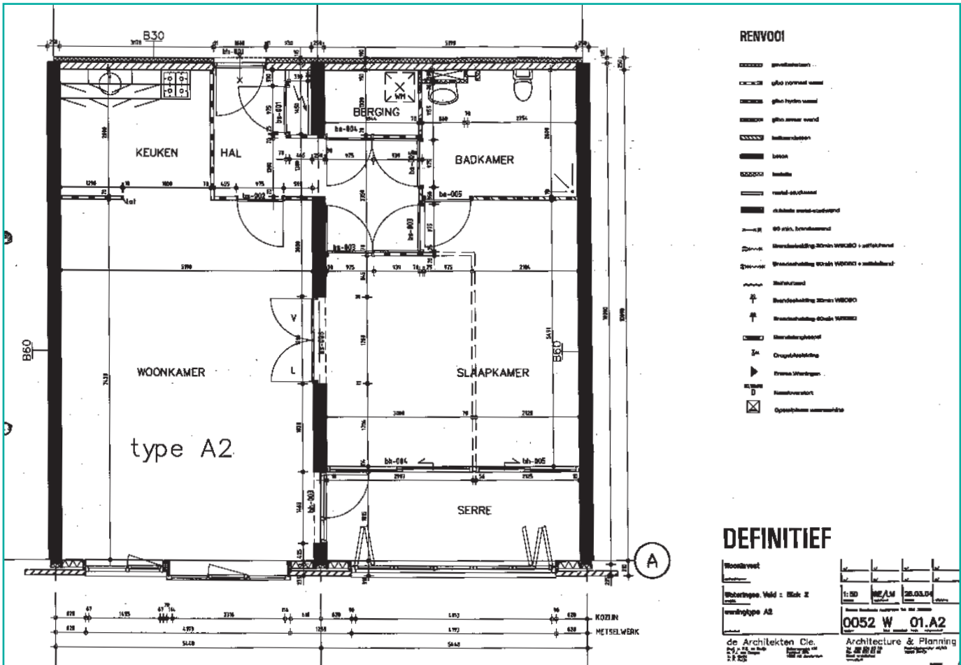
Plattegrond 2-kamerappartement
